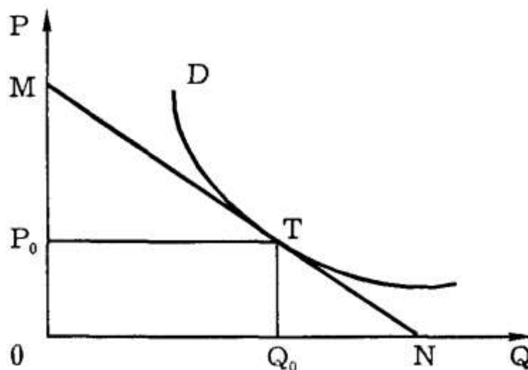
Рис. 3—21. Точечная эластичность
